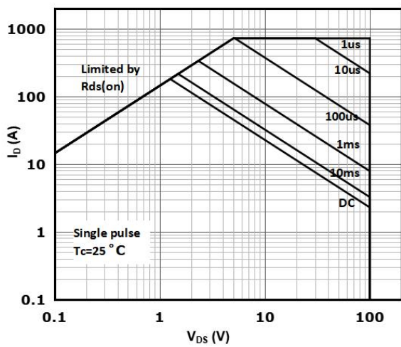
Fig 10 SOA
