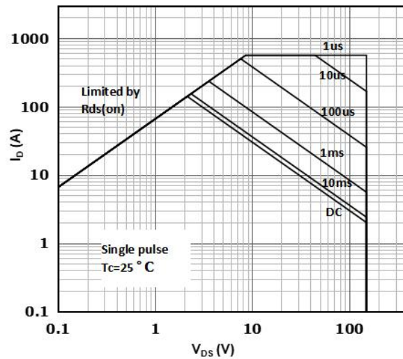
Fig 9 SOA
